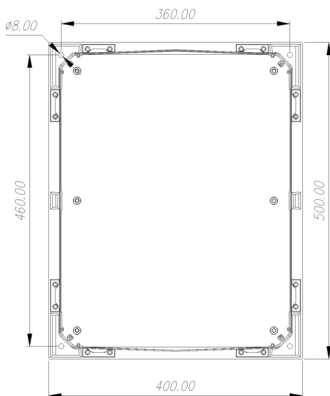
Рисунок 7.2 - Разметка крепления
