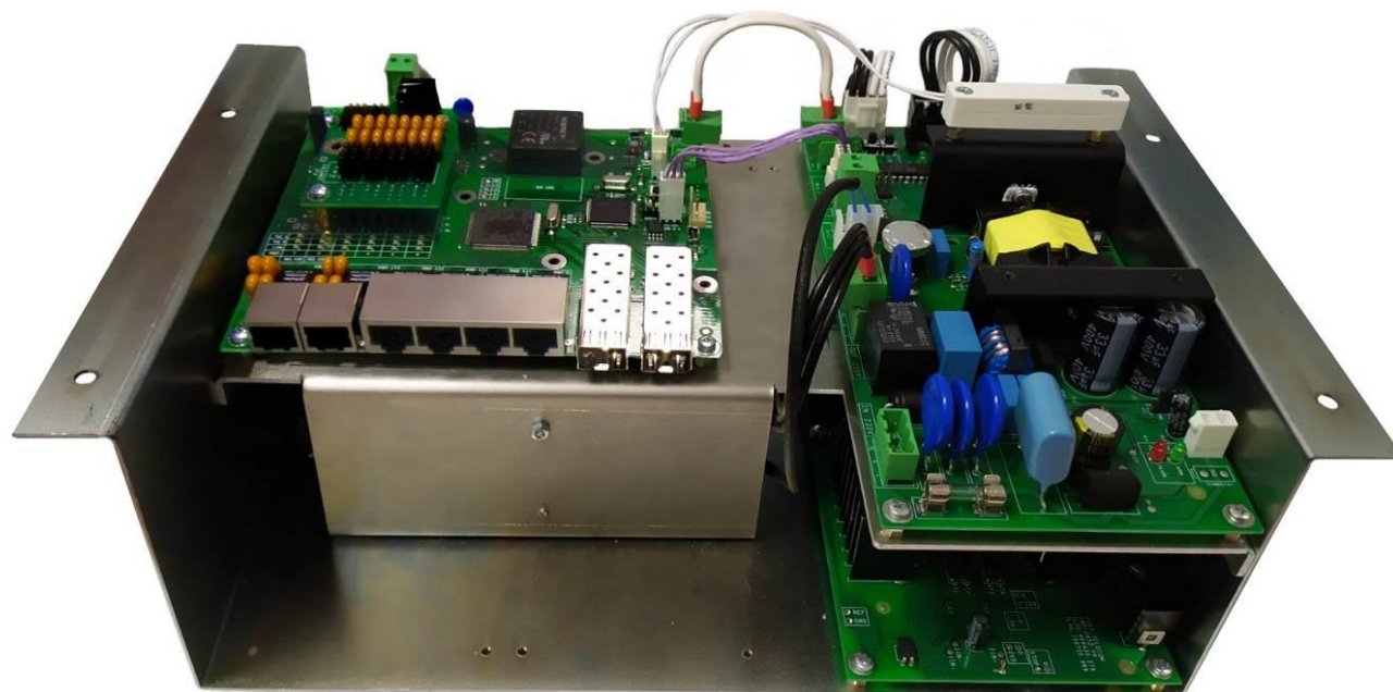
Рисунок 3.4.1 - Платы коммутатора и блоков питания
