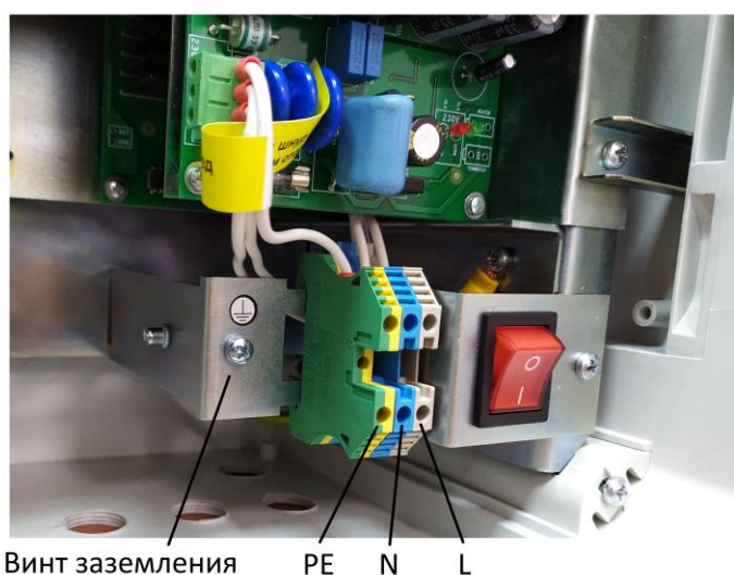
Рисунок 3.5.1 – Узел подключения питания.
