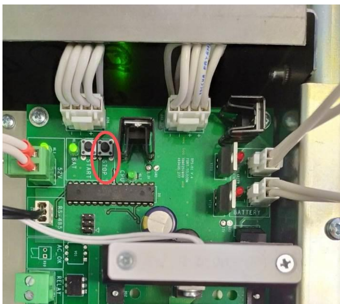
Рисунок 3.5.4 – Нажмите кнопку STOP для отключения питания от АКБ.
